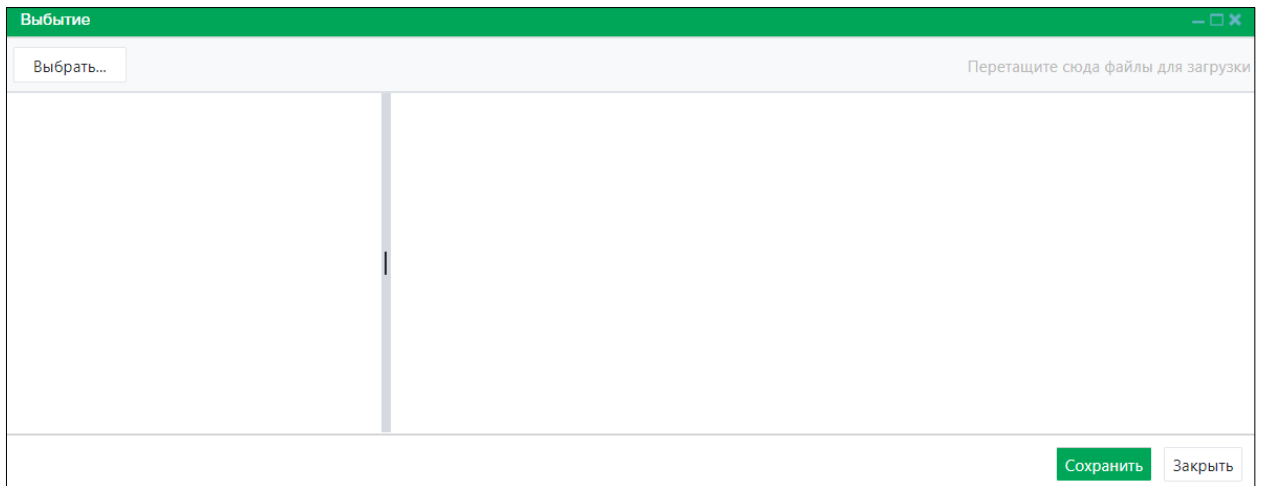
Рисунок 73. Окно «Выбытие»
